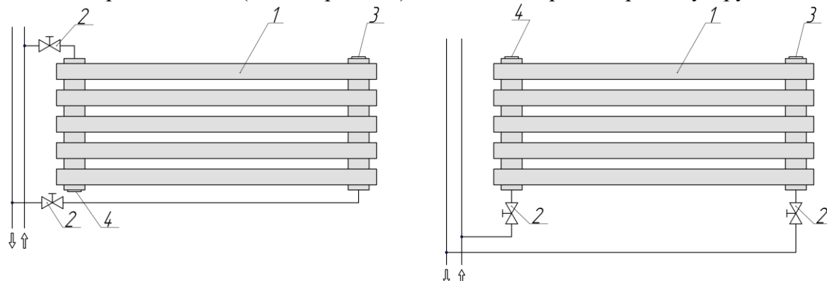
Рис. 3 1. Радиатор. 2. Вентиль (кран). 3. Кран-воздухоотводчик. 4. Пробка глухая.
